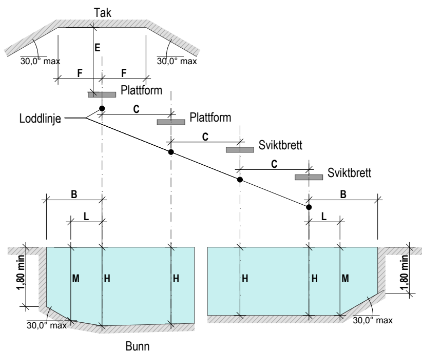
LENGDESNITT
