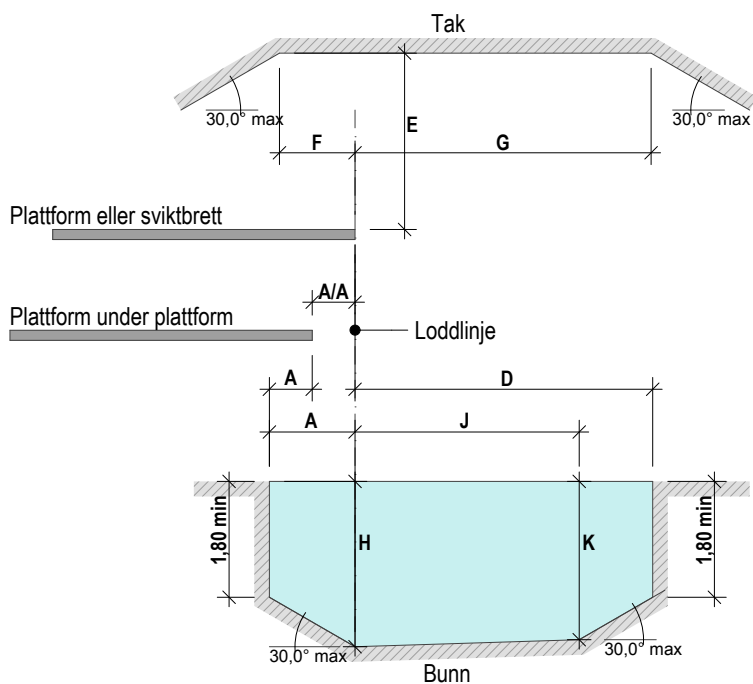
LENGDESNITT
