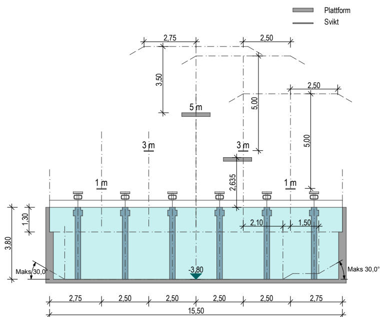
Tversnitt
