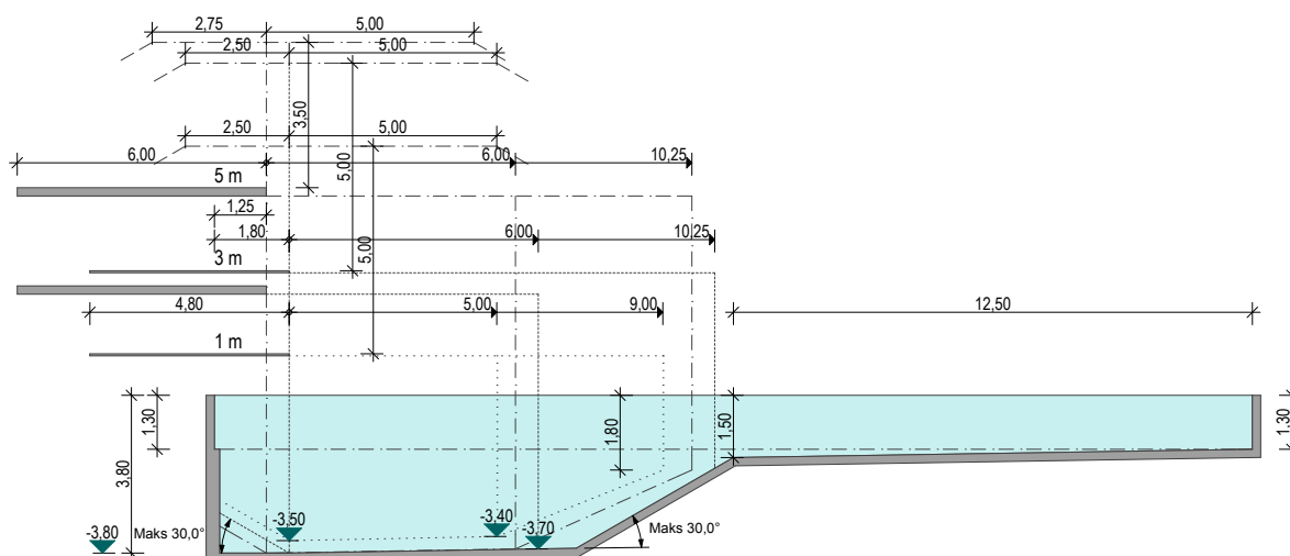
Lengdesnitt
